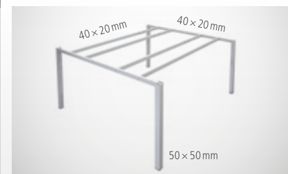
Zdvojená podnož je základem pro dvě protilehlá pracovní místa. Platí také pro UNI A a UNI O.
