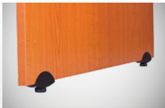
Rektifikace slouží k dorovnání nerovností podlahy až o 1,5cm
