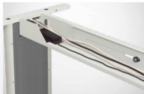
Kabelový kanál poskytuje prostor pro vedení kabelů a uložení elektroinstalace
